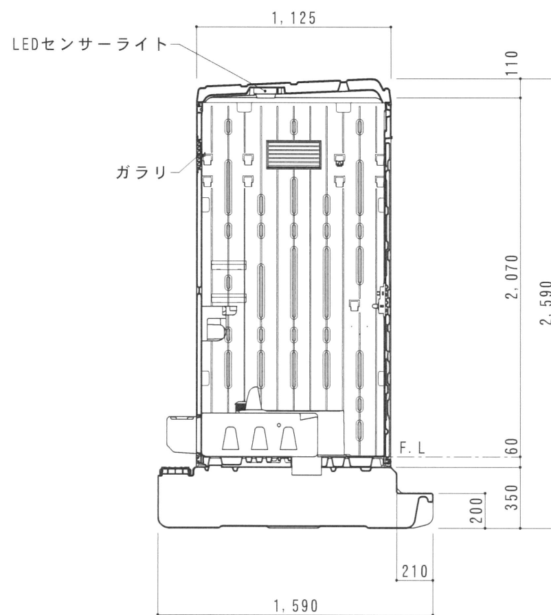
断面図 S=1/30
