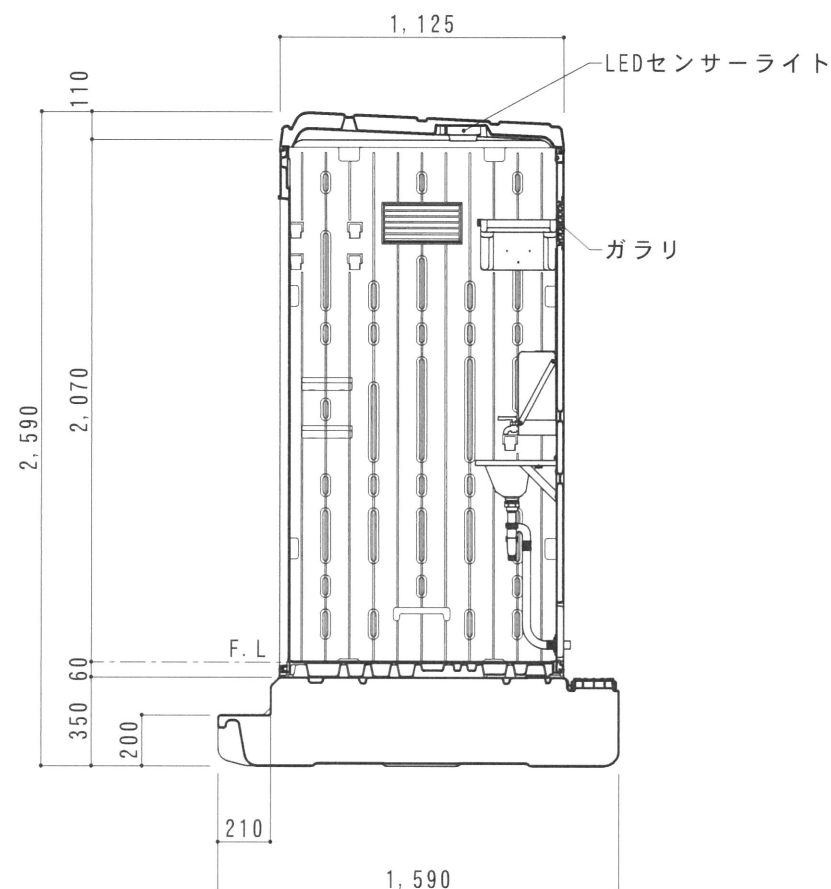
断面図 S=1/30
