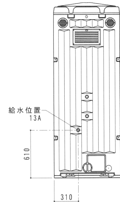
C 立面图 S=1/30
