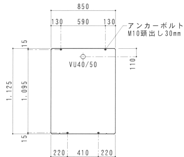
土台底面図 S=1/30
