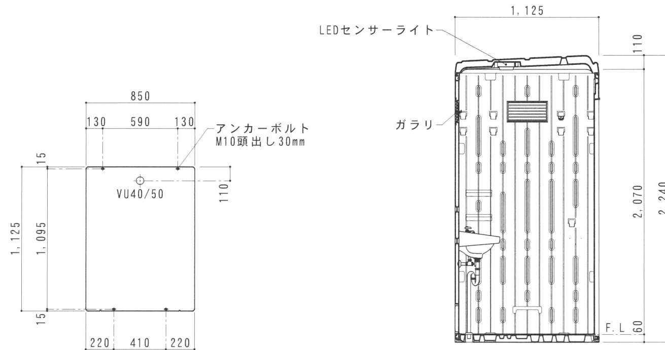
断面図 S=1/30
