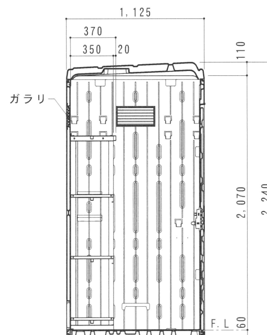
断面図 S=1/30
