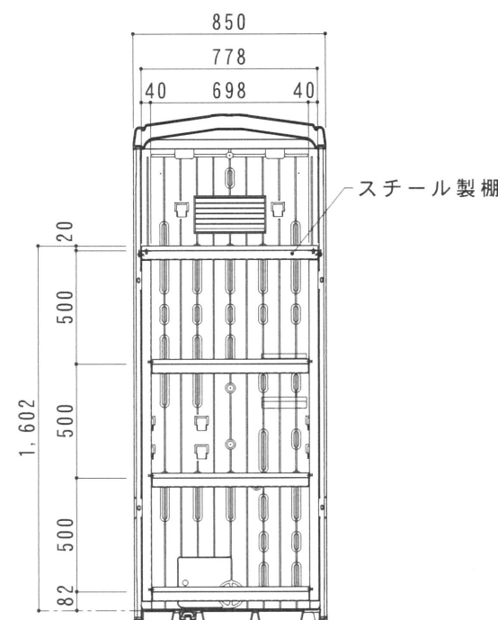
断面図 S=1/30
