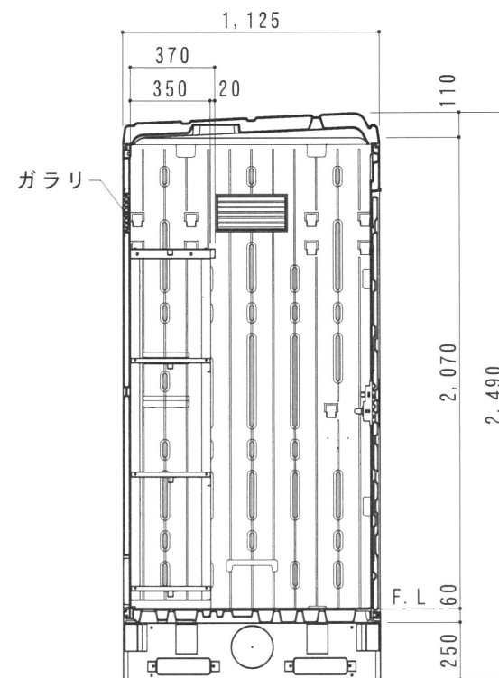
断面図 S=1/30
