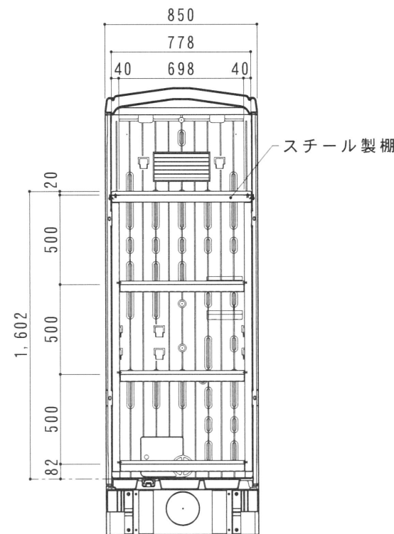
断面図 S=1/30
