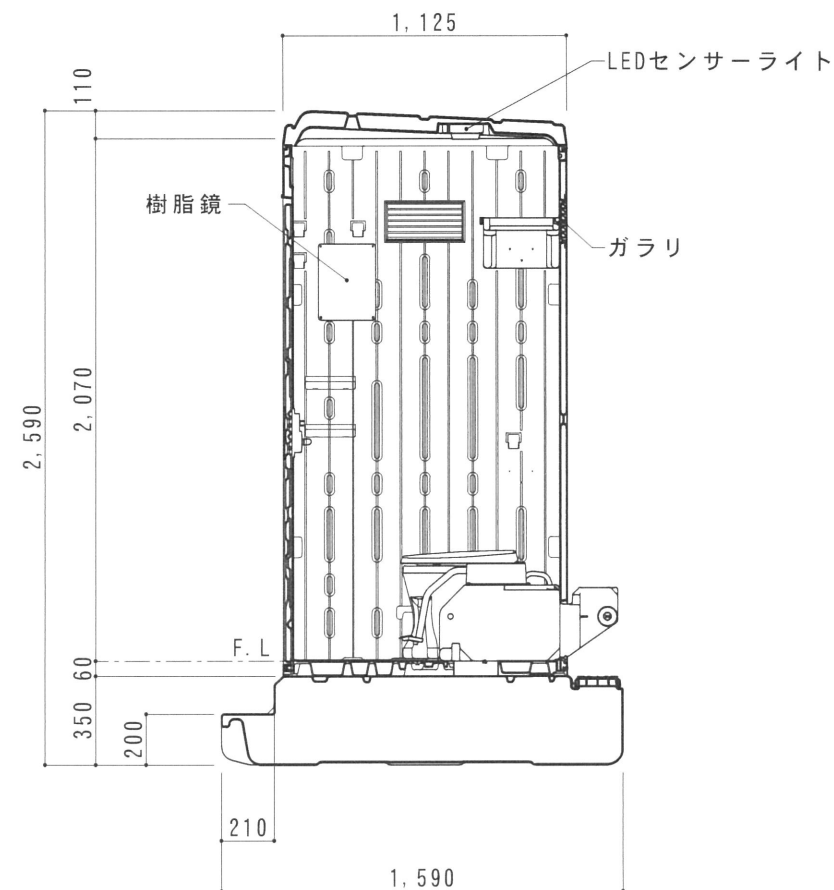
断面図 S=1/30
