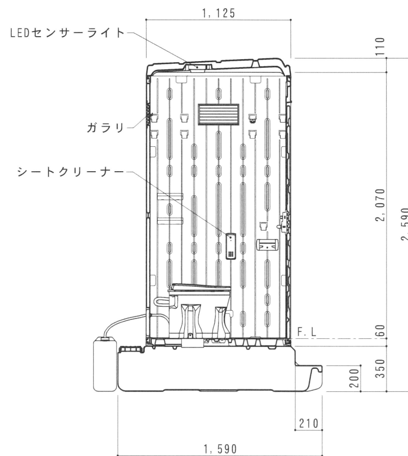
断面図 S=1/30
