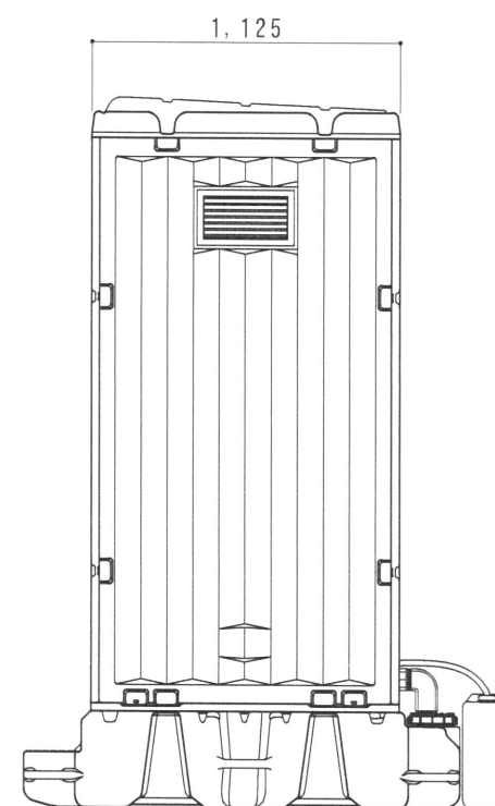
D 立面図 S=1/30
