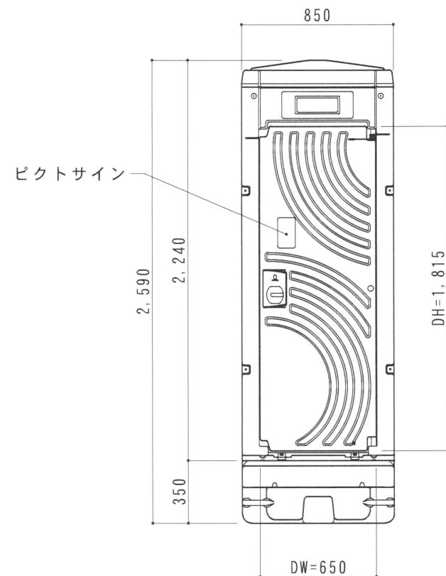
A 立面図 S=1/30
