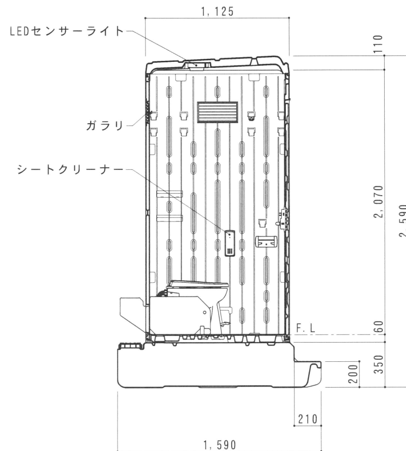
断面図 S=1/30
