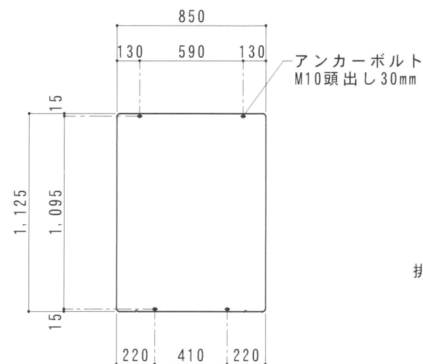
土 台 図 S=1/30
