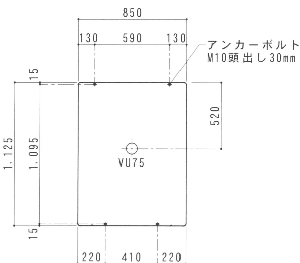
土台底面図 S=1/30
