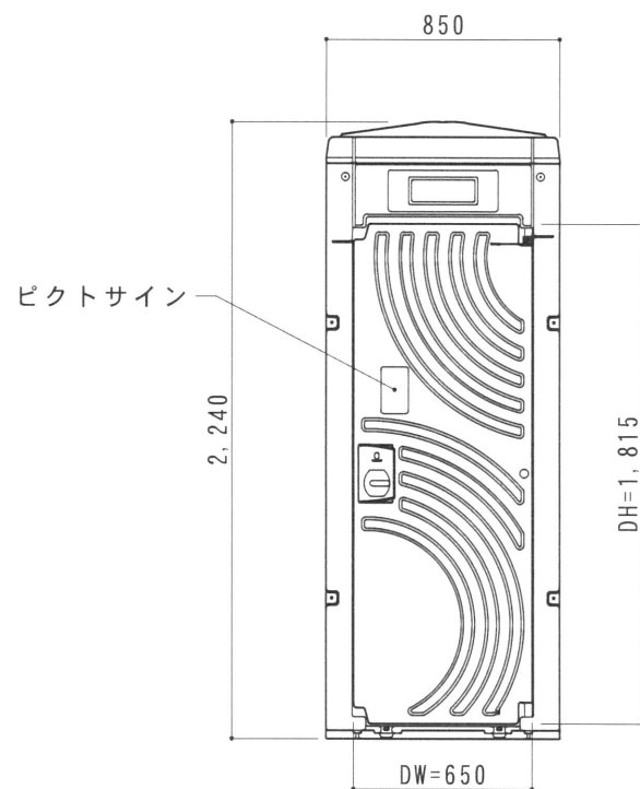
A 立面図 S=1/30
