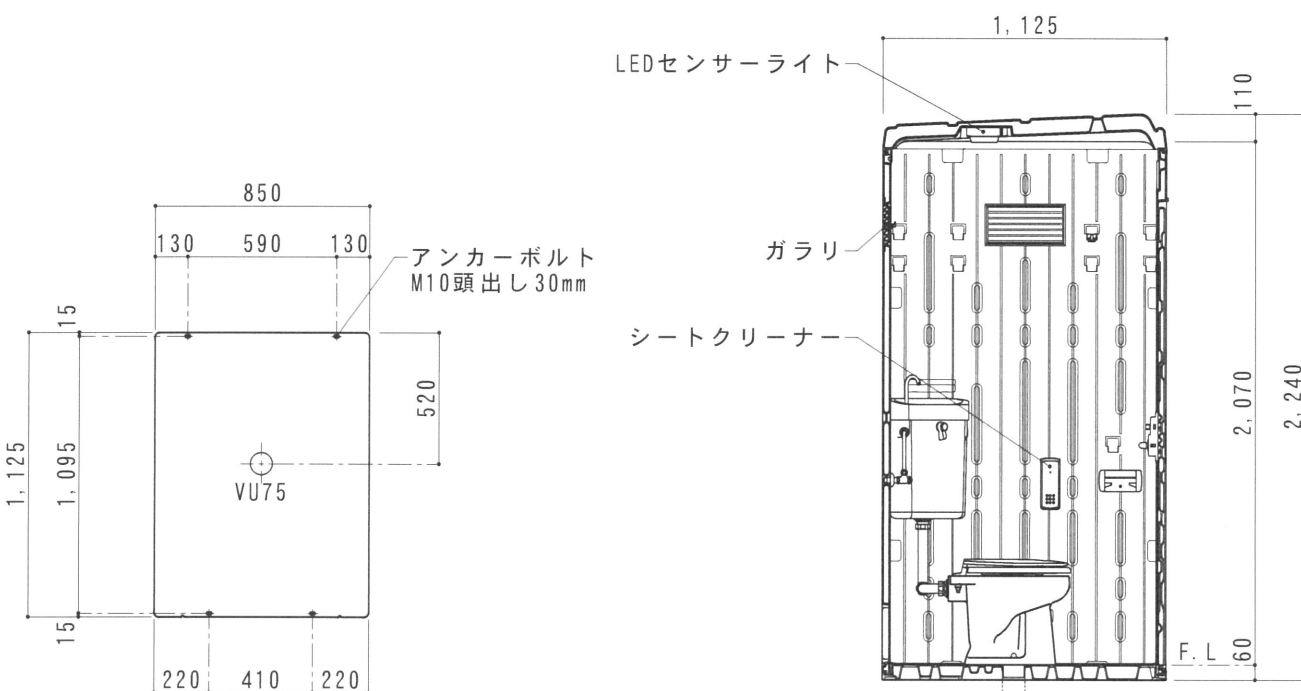
断面図 S=1/30
