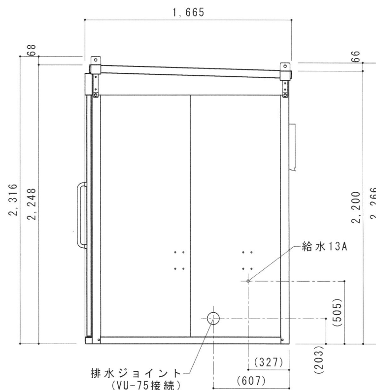
D 立面図 S=1/30
