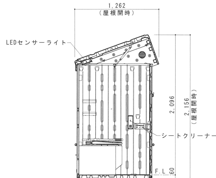
断面図 S=1/30
