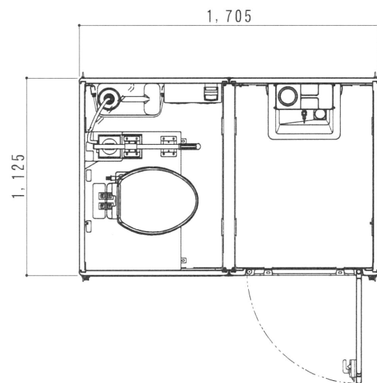
平面図 S=1/30
