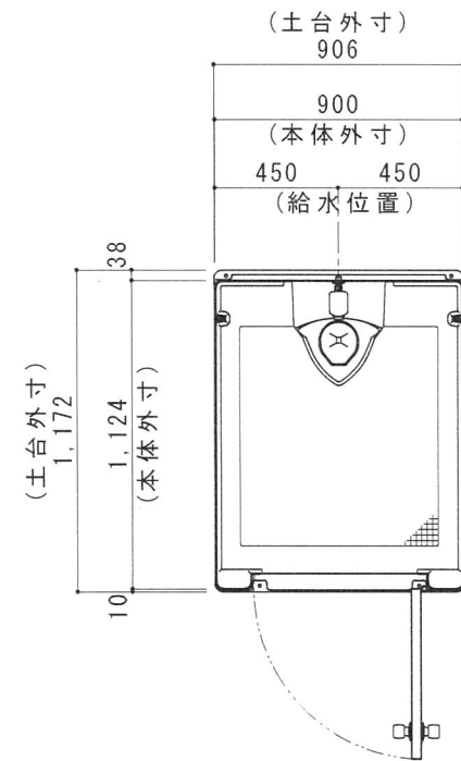
平面図 S=1/30
