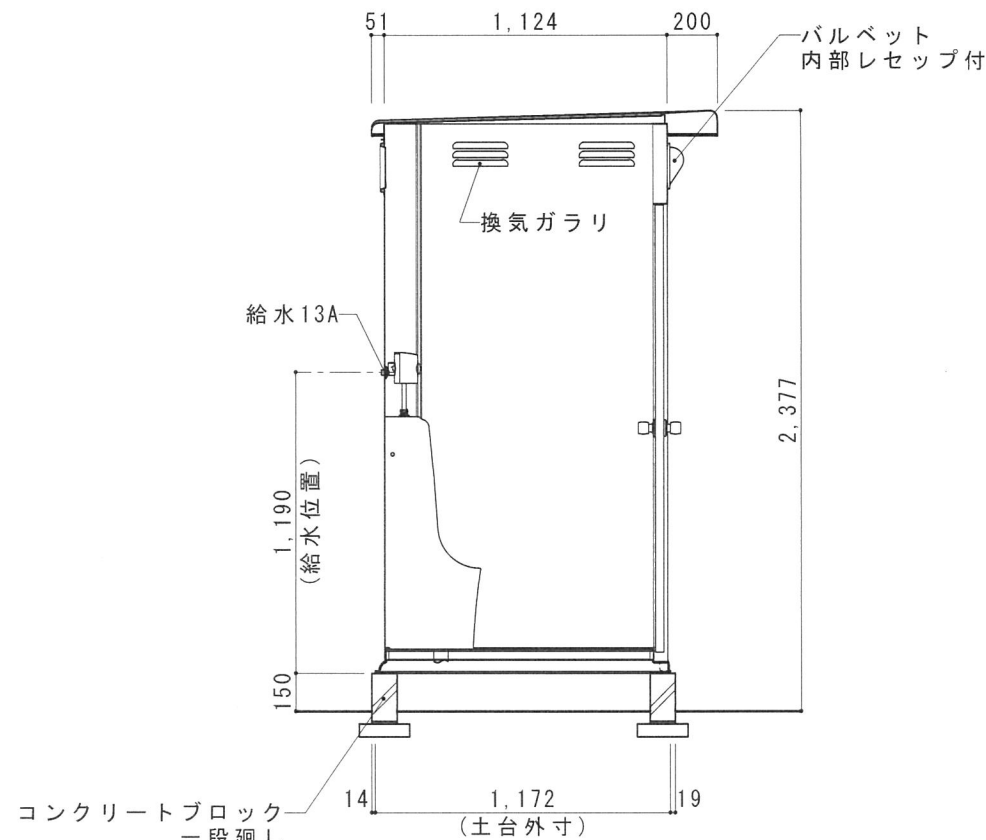
断面図 S=1/30
