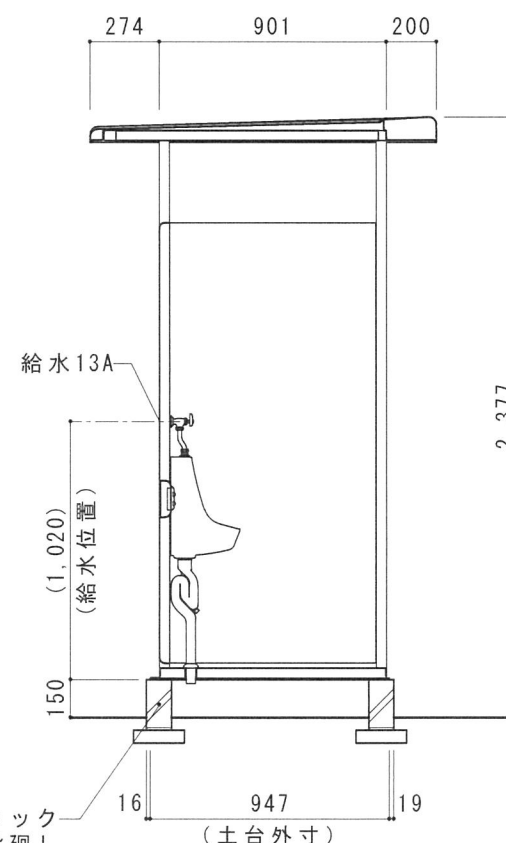
断面图 S=1/30
