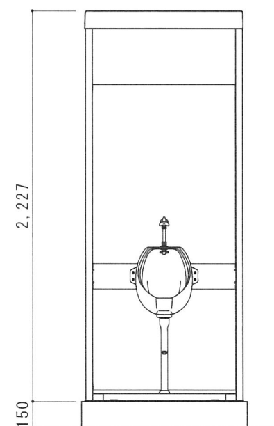
A 立面图 S=1/30
