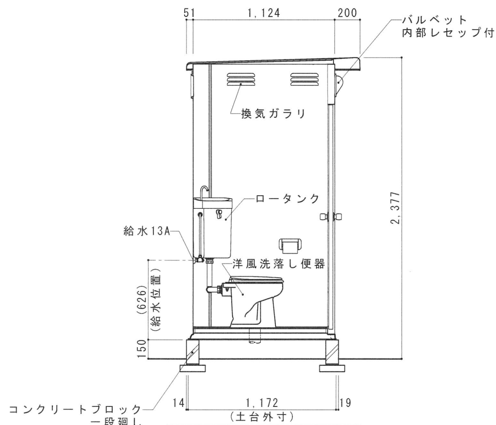
断面図 S=1/30
