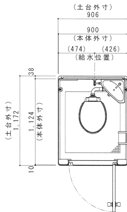
平面図 S=1/30
