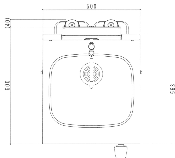
平面図 S=1/10
