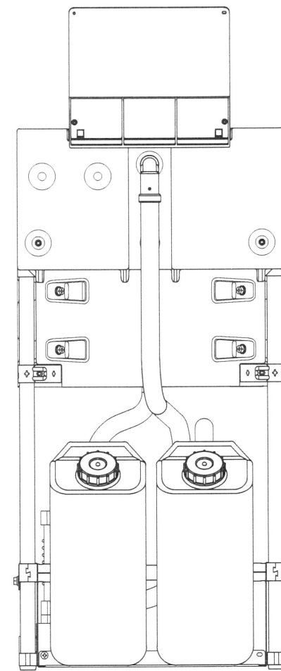
C 立面図 S=1/10
