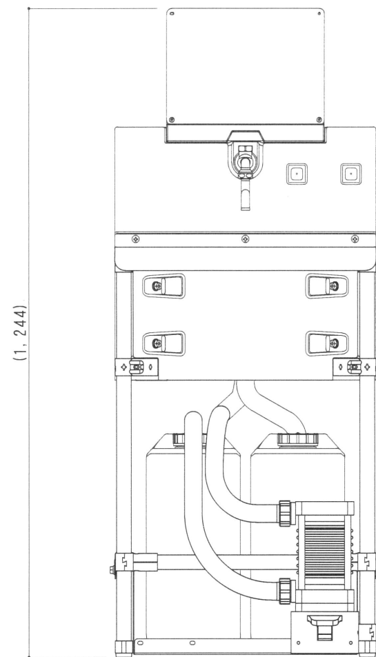
A 立面図 S=1/10
