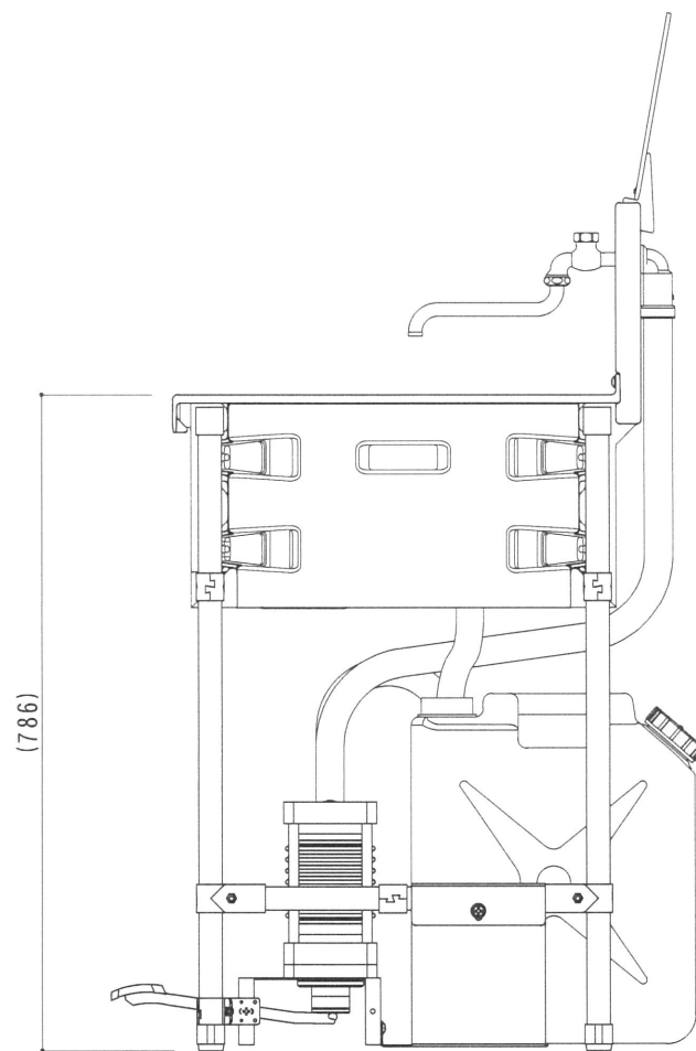
D 立面図 S=1/10
