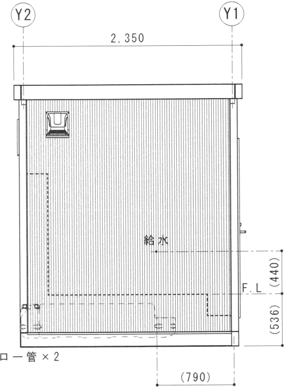
B 立面図 S=1/40
