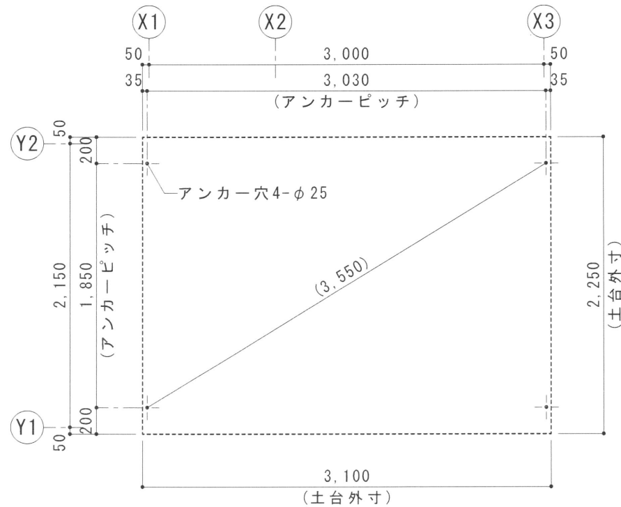
アンカー位置図 S=1/40
