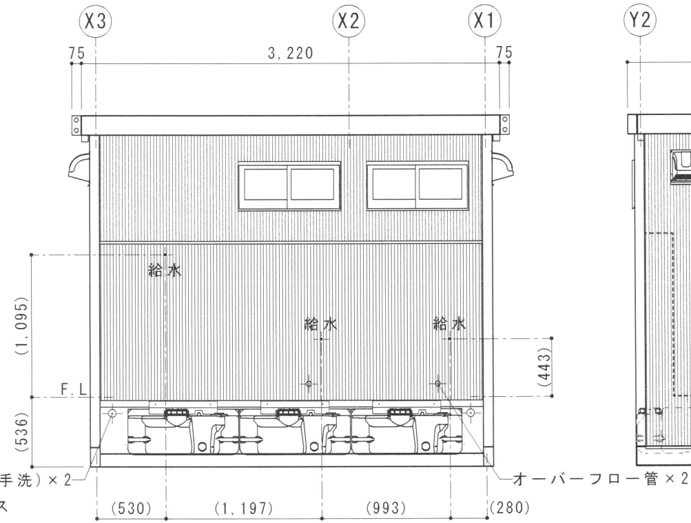
C 立面図 S=1/40 手排水: VU50 給水: HIVP13
