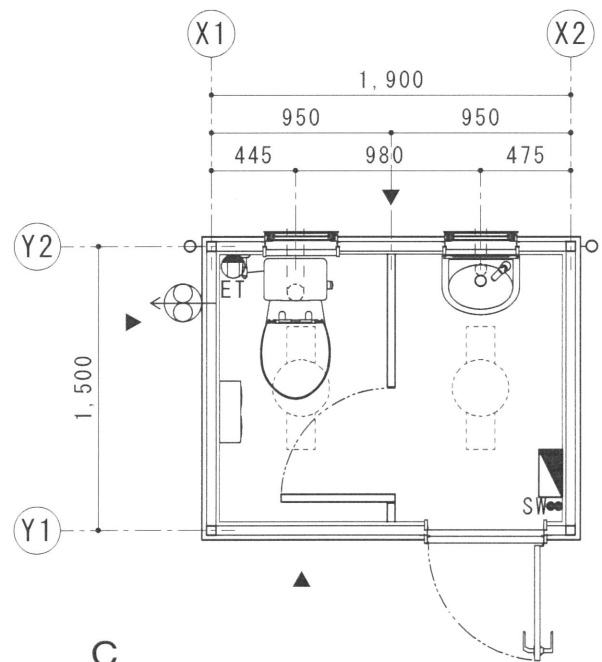
平面図 S=1/40 ▲ブレース位置
