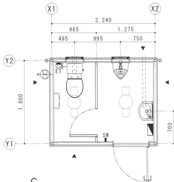
平面図 S=1/40
