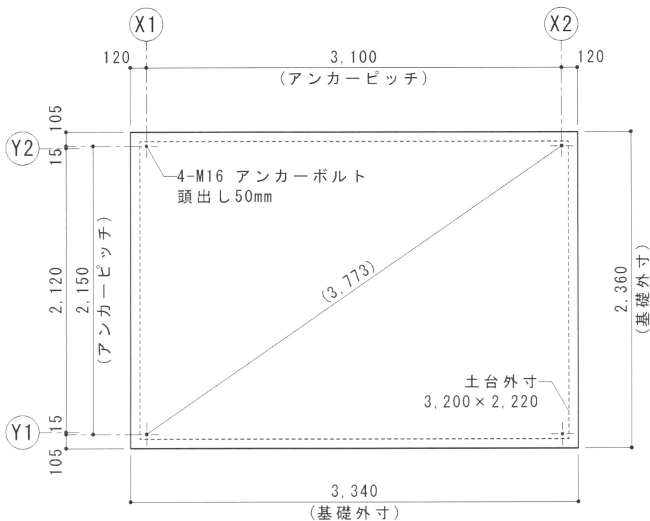
参考基礎図 S=1/40
