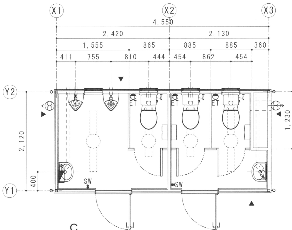
平面図 S=1/50 ▲ブレース位置
