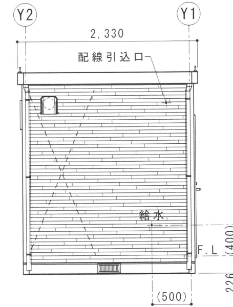
B 立面図 S=1/50
