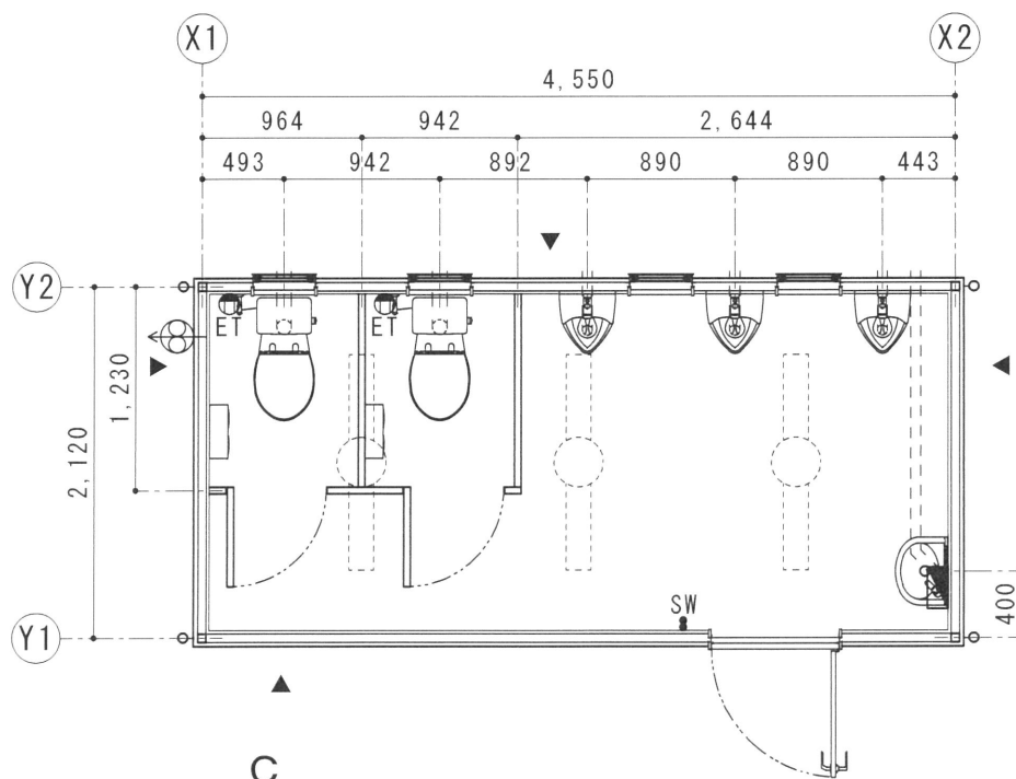
平面図 S=1/50
