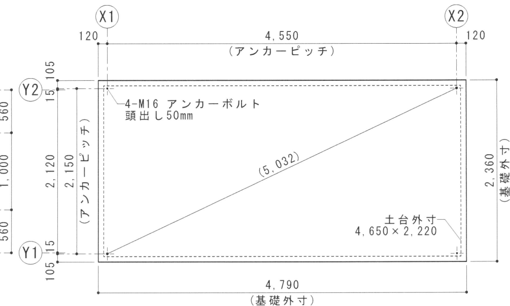
参考基礎図 S=1/50
