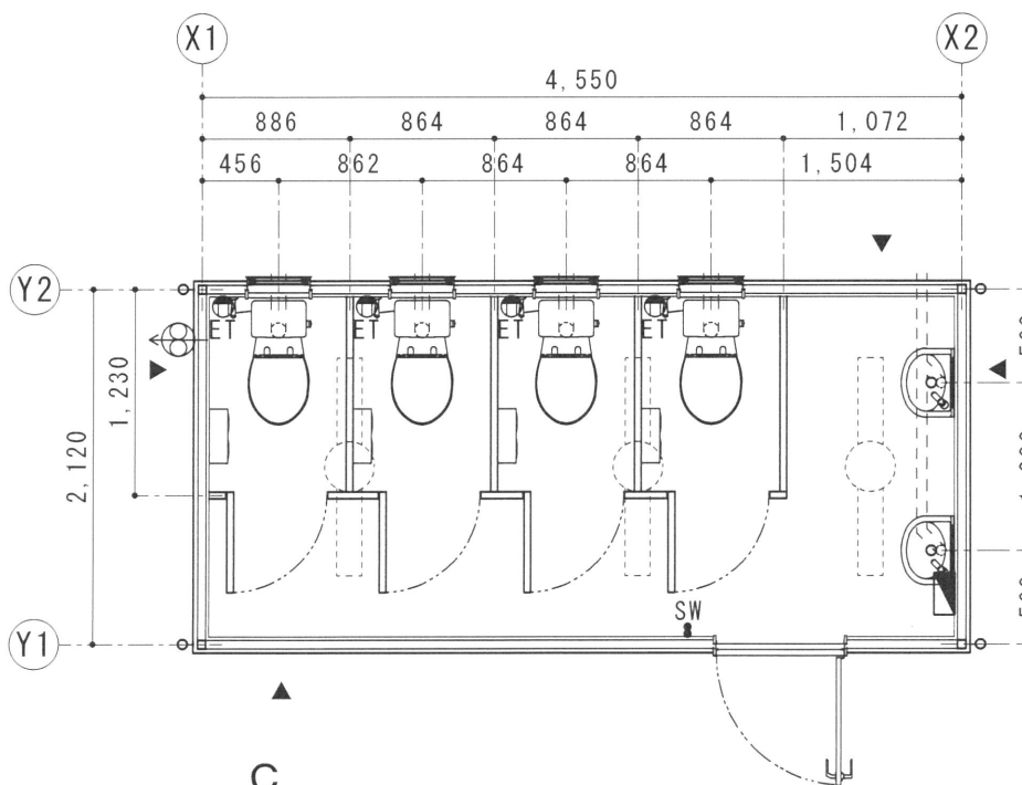
平面図 S=1/50
