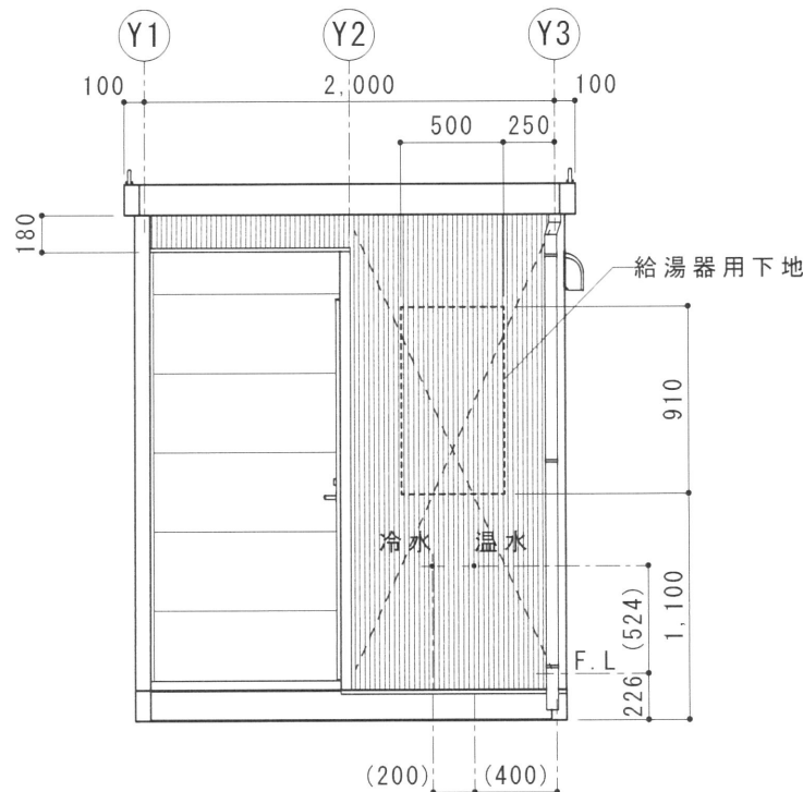
D 立面図 S=1/40
