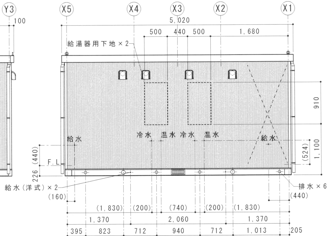
C 立面図 S=1/50
