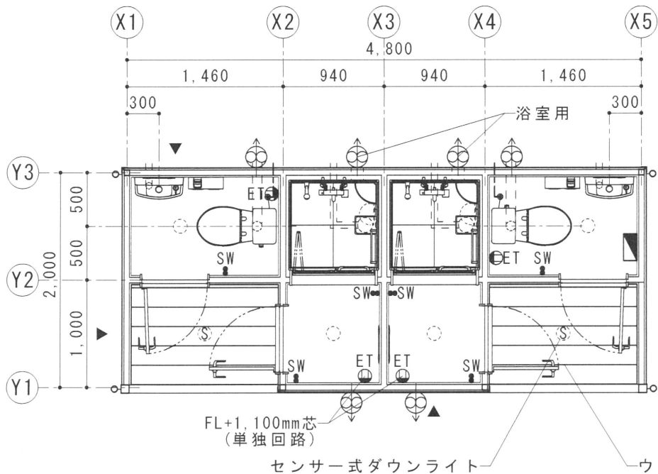
平面図 S=1/50
