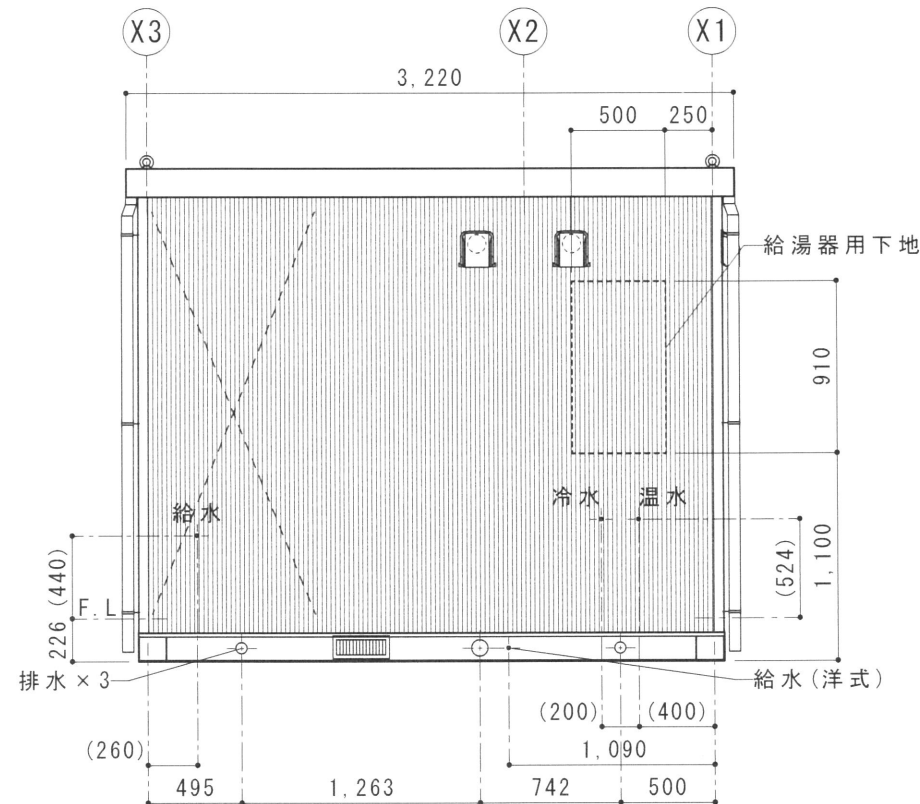
C 立面図 S=1/40
