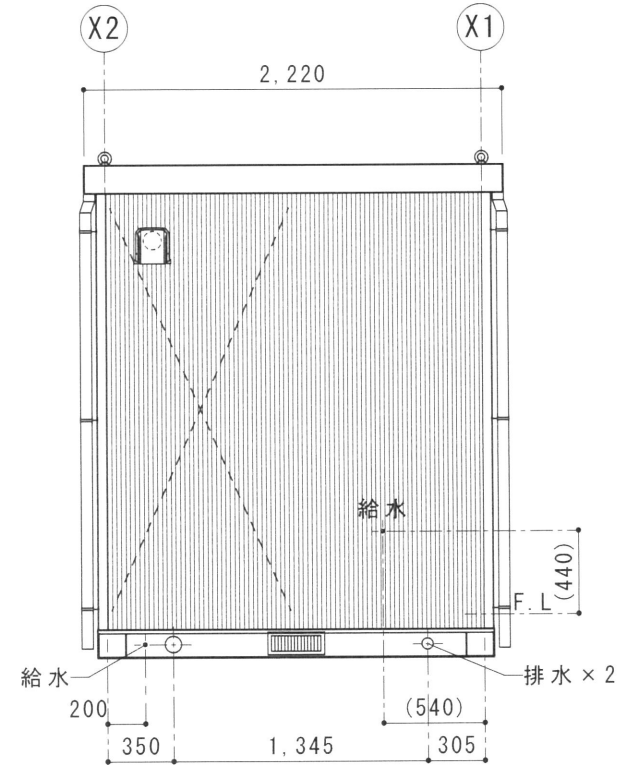
C 立面図 S=1/40
