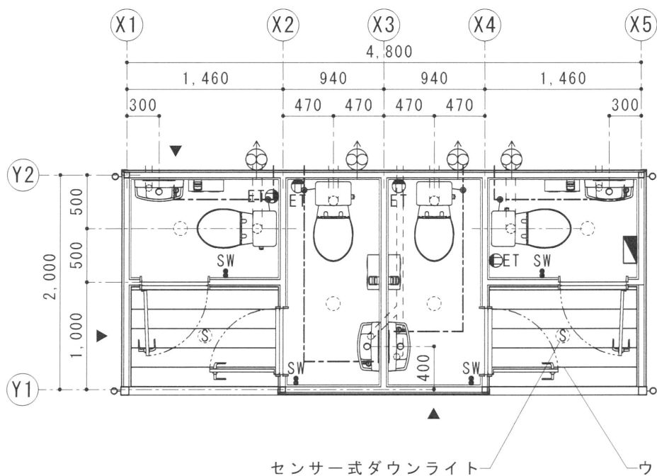
平面図 S=1/50
