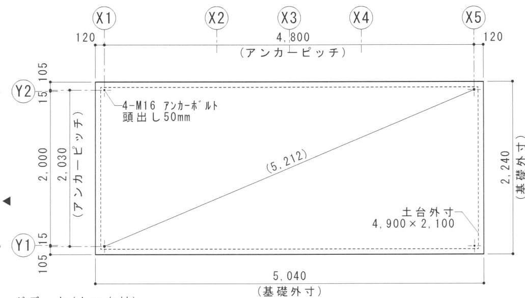
参考基礎図 S=1/50
