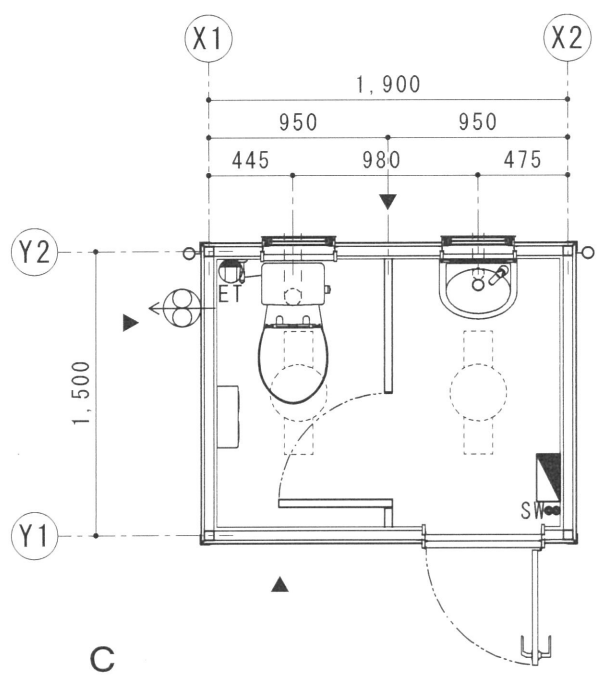
平面図 S=1/40 ▲ブレース位置
