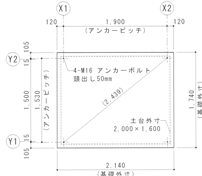
参考基礎図 S=1/40 ベタ基礎は別途工事
