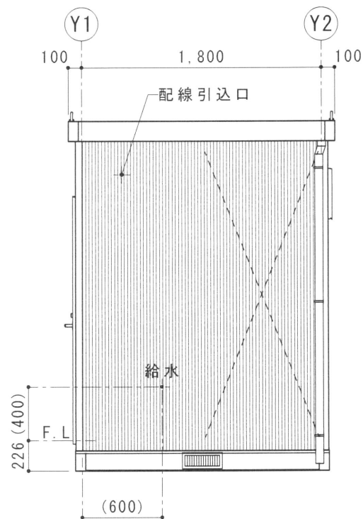
D 立面図 S=1/40
