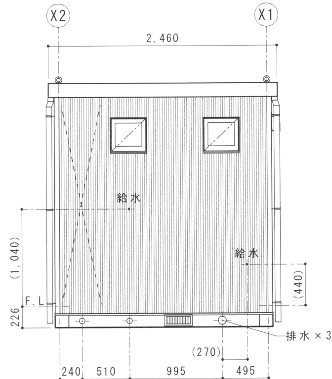
C 立面図 S=1/40
