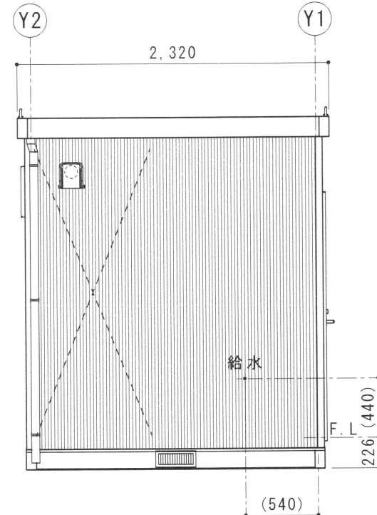
B 立面図 S=1/40
