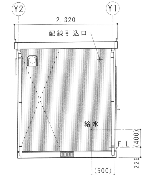
B 立面図 S=1/50
