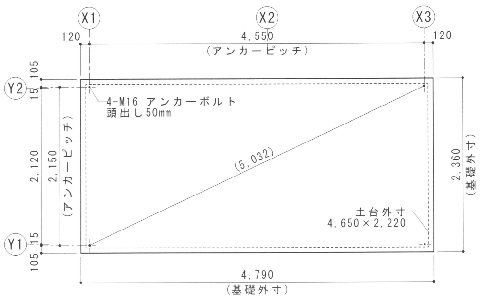
参考基礎図 S=1/50 ベタ基礎は別途工事
