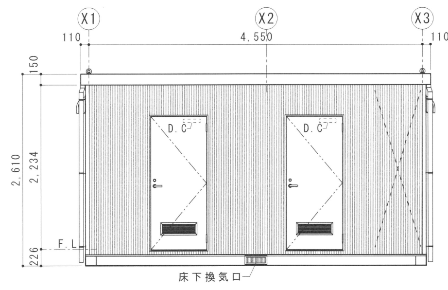
A 立面図 S=1/50
