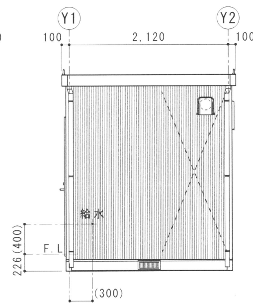
D 立面図 S=1/50
