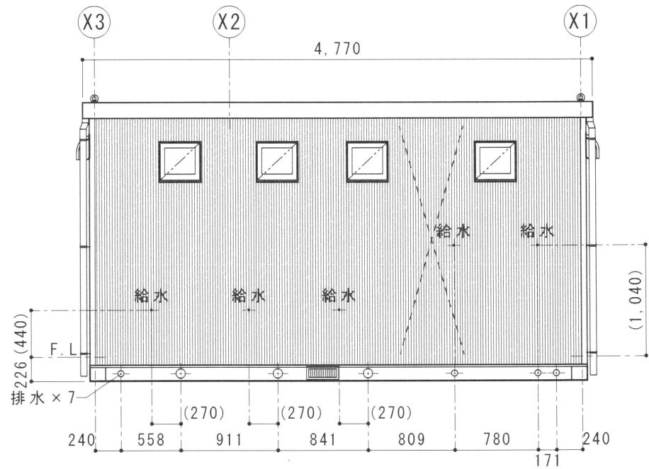
C 立面図 S=1/50 大排水: VU75 小・手排水: VU50 給水: HIVPi3
