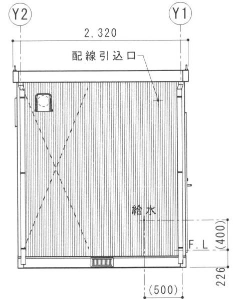
B 立面図 S=1/50
