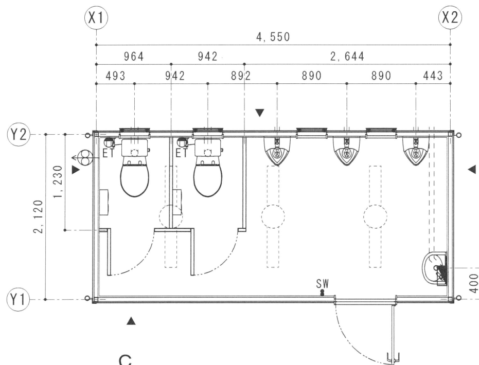
平面図 S=1/50
