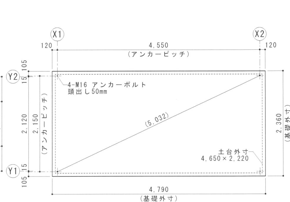
参考基礎図 S=1/50
