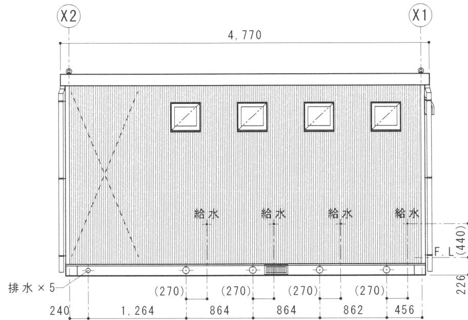
C 立面図 S=1/50
