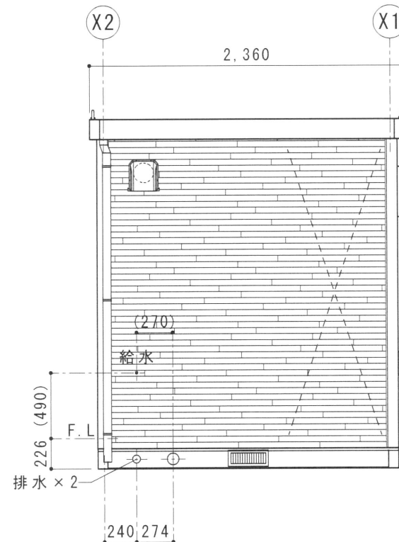
C 立面図 S=1/40
