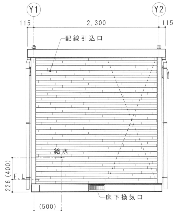
D 立面図 S=1/40
