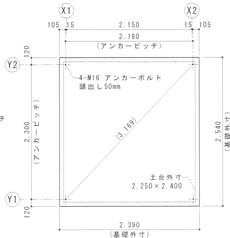
参考基礎図 S=1/40
