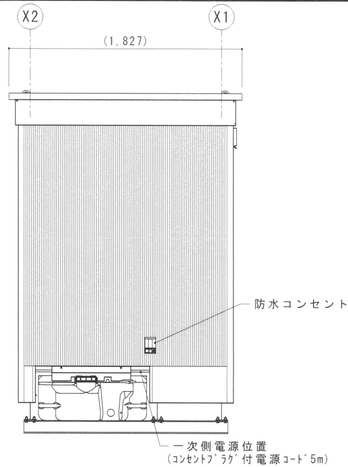
C 立面図 S=1/30
