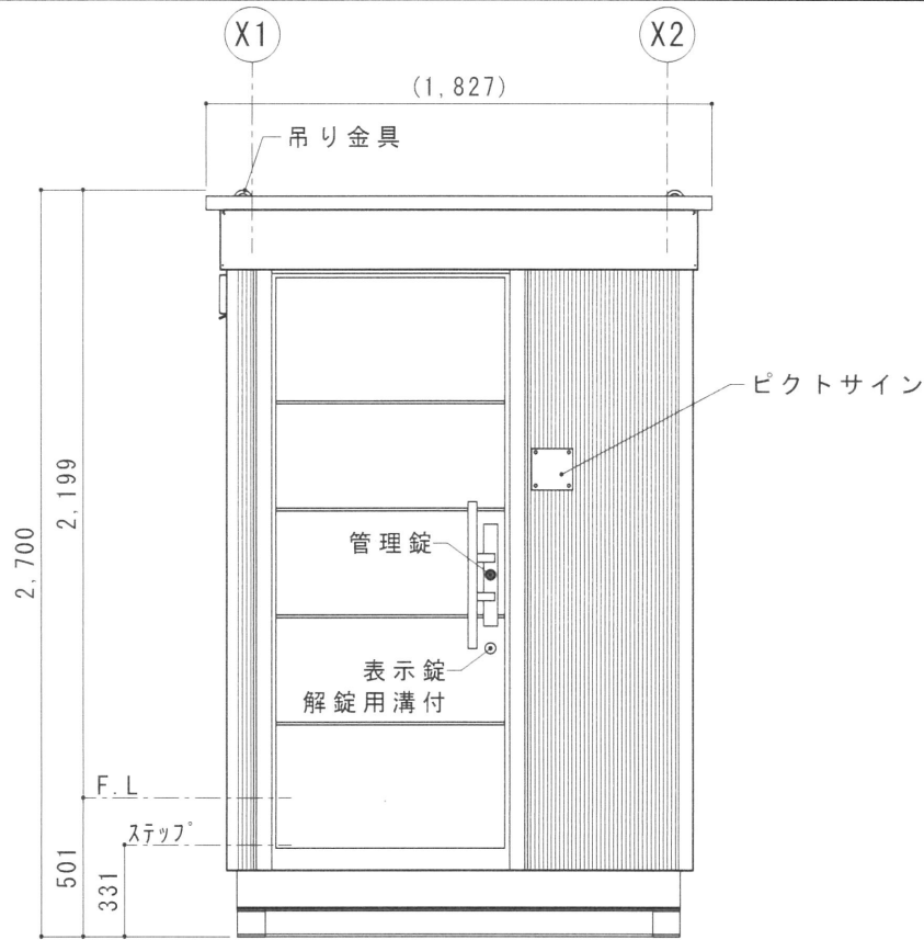
A 立面図 S=1/30
