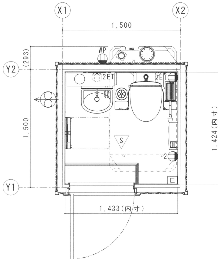
平面図 S=1/30
