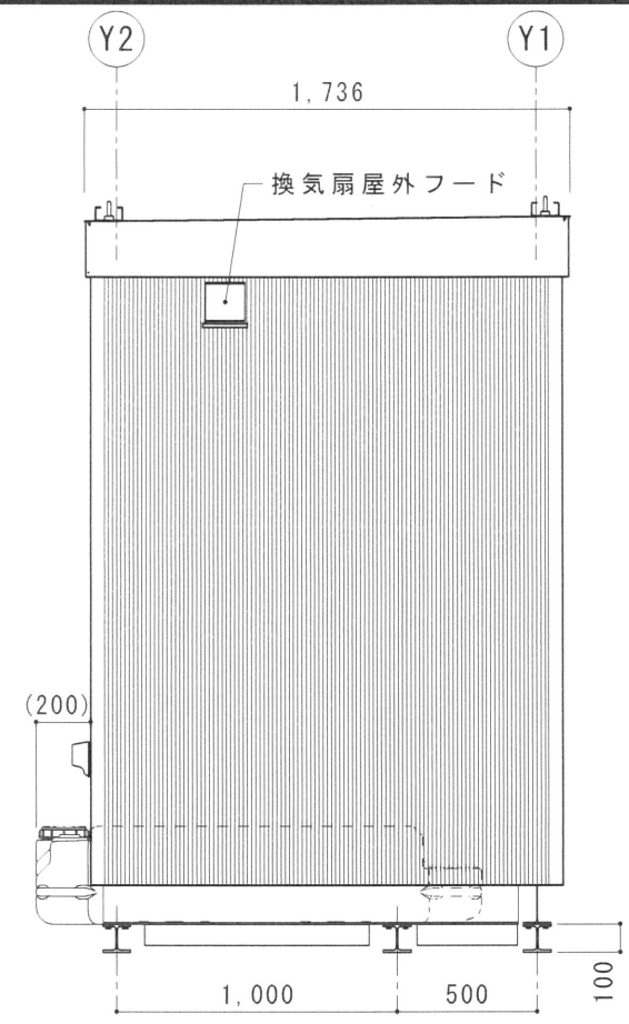
B 立面図 S=1/30
