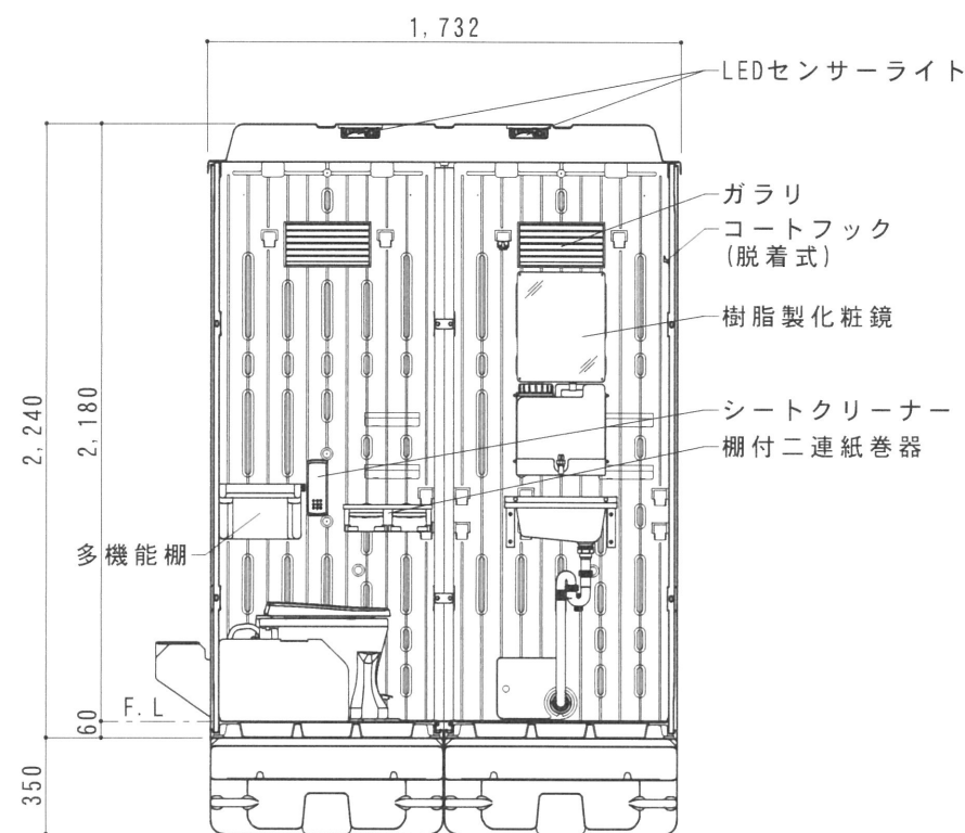
断面図 S=1/30
