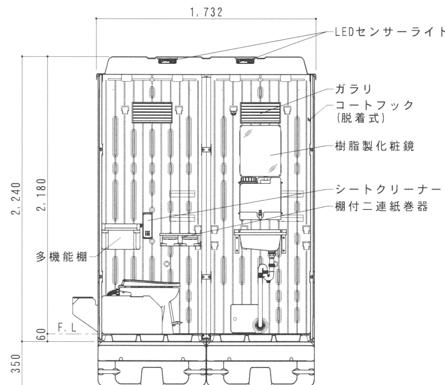
断面図 S=1/30
